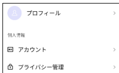
設定画面
